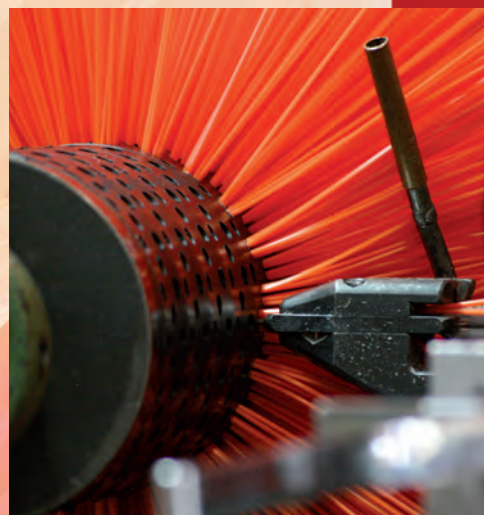
Perforado en espiguilla en V cerrado
